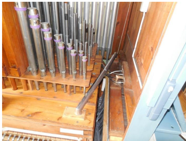
Piber på vindlade. Tinkondukt
